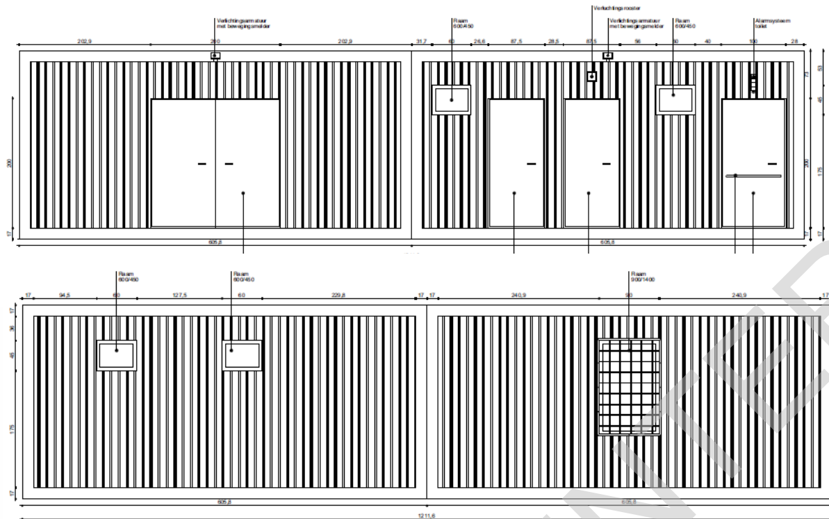
AANZICHT 2
