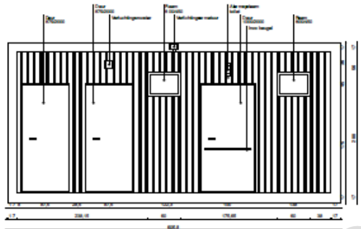
AANZICHT 1
